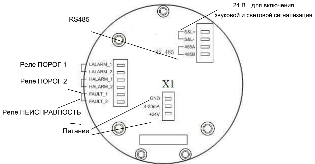
Рис. 3. Плата газоанализатора
